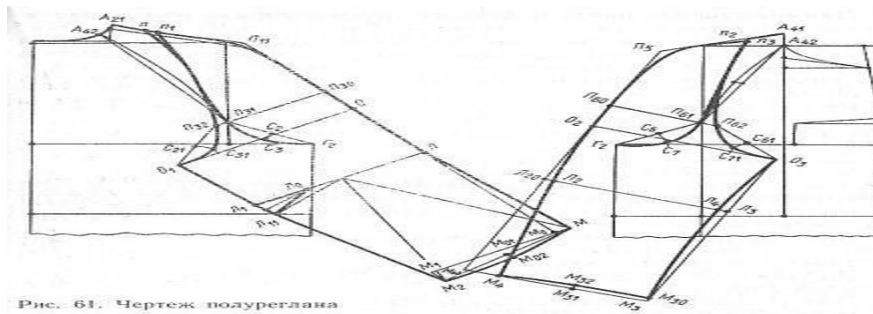
Рис. 61. Чертеж полуреглана
