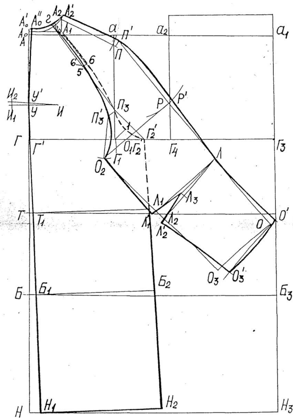
Рис. 8.3 Чертеж конструкции задней части рукава покроя реглан
