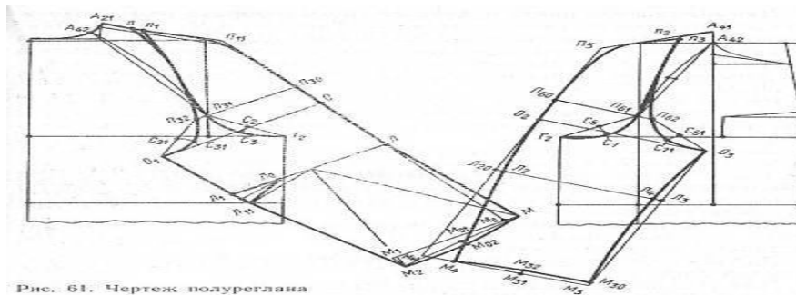
Рис. 61. Чертеж полуреглана
