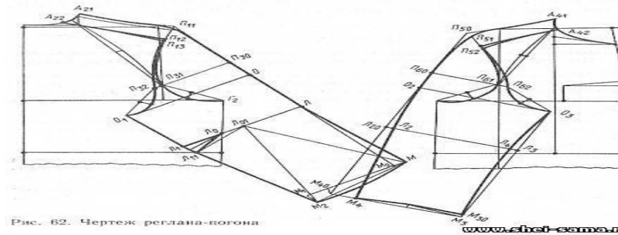
Рис. 8.5 Чертеж конструкции передней и задней части рукава покроя реглан-погон
