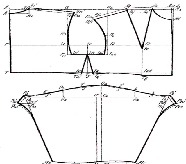
Рис. 7.3 Чертеж конструкции рукава с квадратной проймой
