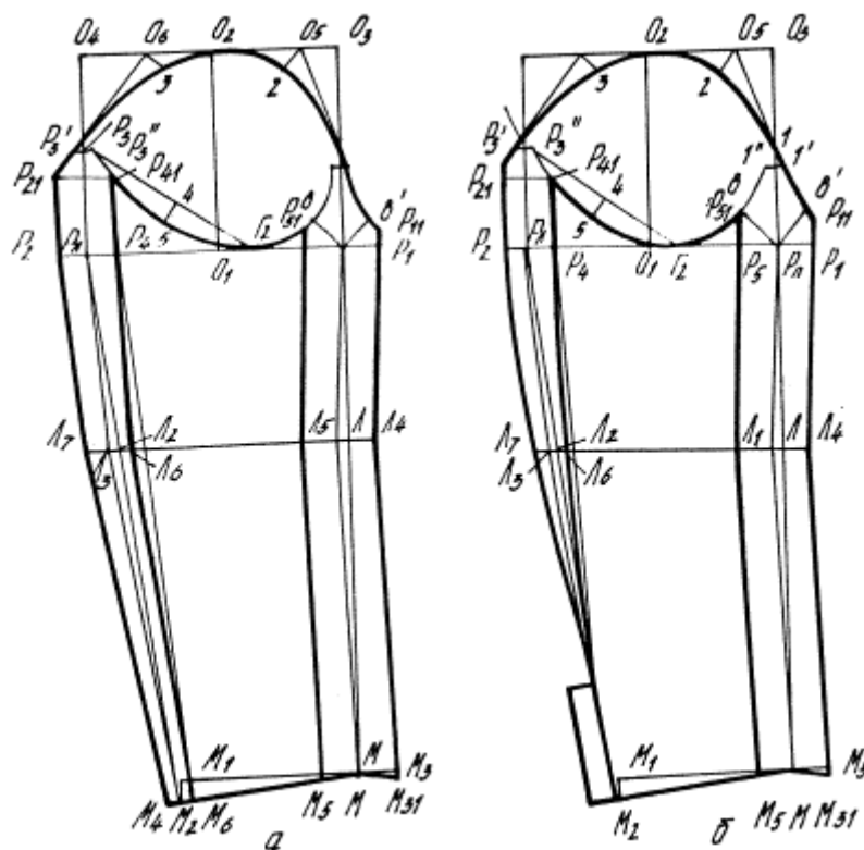
Рис. 5.3. Варианты конструкции двухшовного рукава
