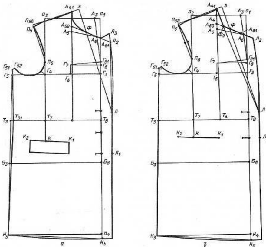
Рис. 42. Чертеж борта и лацкана однобортного пальто:
