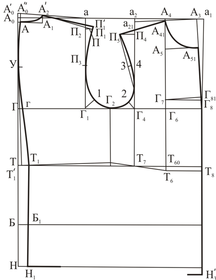
Рис. конструкции пиджака
