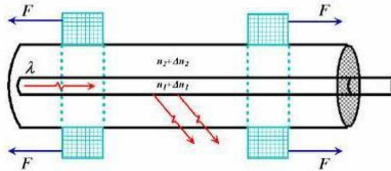
Рис. 12. Формирование канала утечки растяжением оптоволокну при воздействии внешнего усилия F
