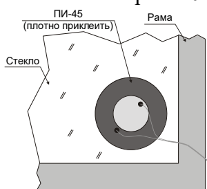
Рисунок 10 – Крепление генераторов-вибровозбудителей "СВ-4Б" на стекло
