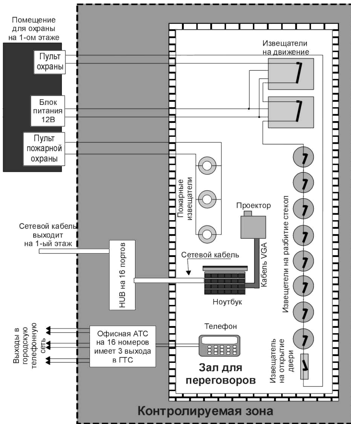
Схема функциональных (сигнальных) цепей
