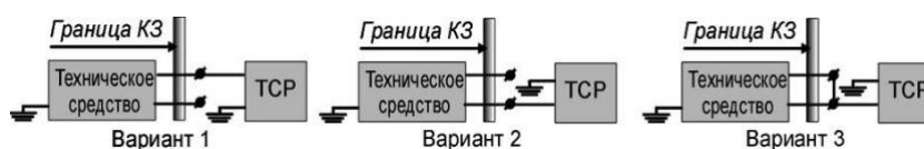
Рис. А2.2. Варианты подключения с использованием цепи Пикара
