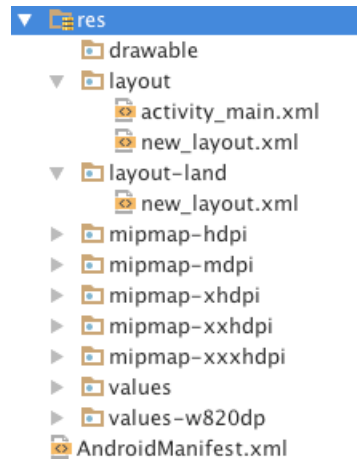
Рис. 5.12. Структура папки ресурсов
