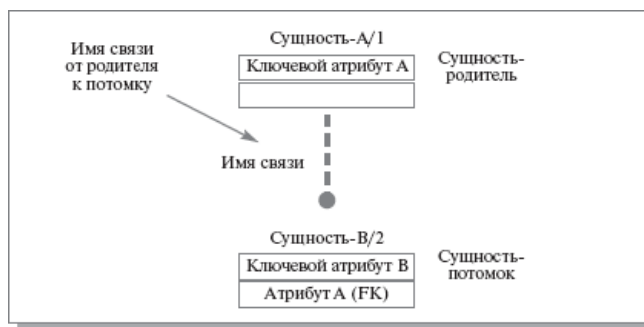
Рисунок 3.4 - Неидентифицирующая связь
