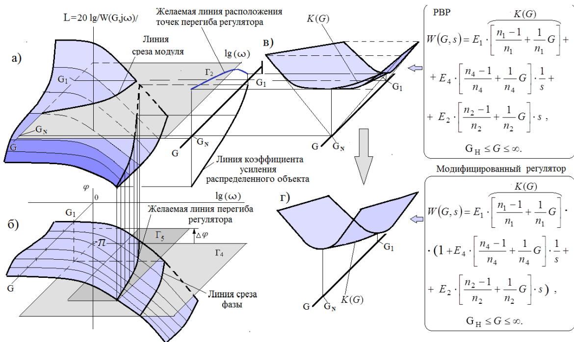
Рис.5. Синтез модифицированного распределенного регулятора
