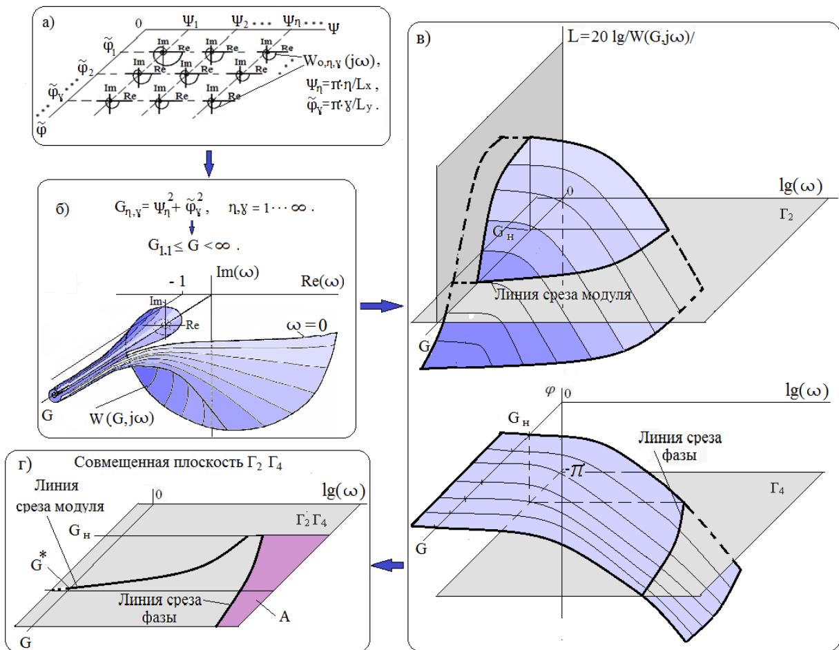
Рис.1. Частотные характеристики распределенного объекта
