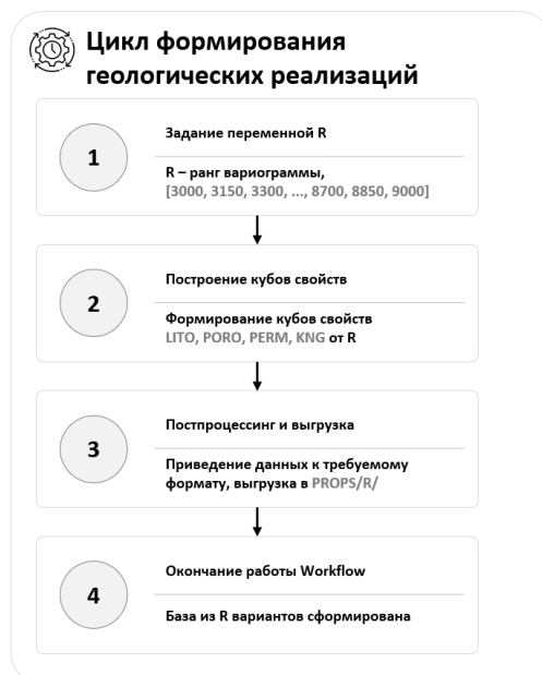
Рисунок 2 – Схема многовариантного геологического моделирования
