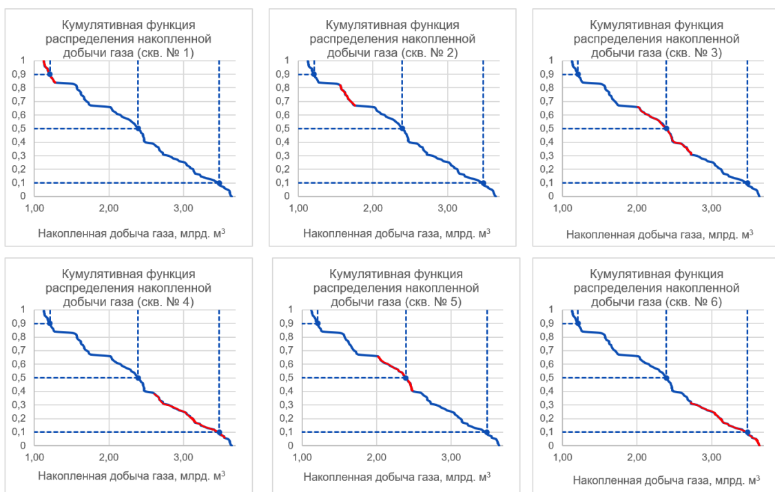
Рисунок 3 – Вероятностный анализ результатов расчета
