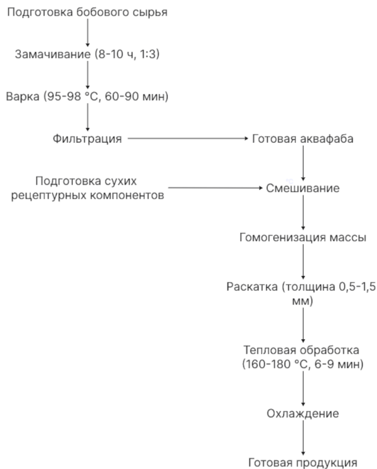
Рисунок 1. Технологическая схема получения снеков на основе аквафабы
