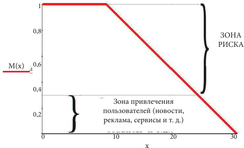
Рис. 3. Оценка риска скорости увеличения трафика
