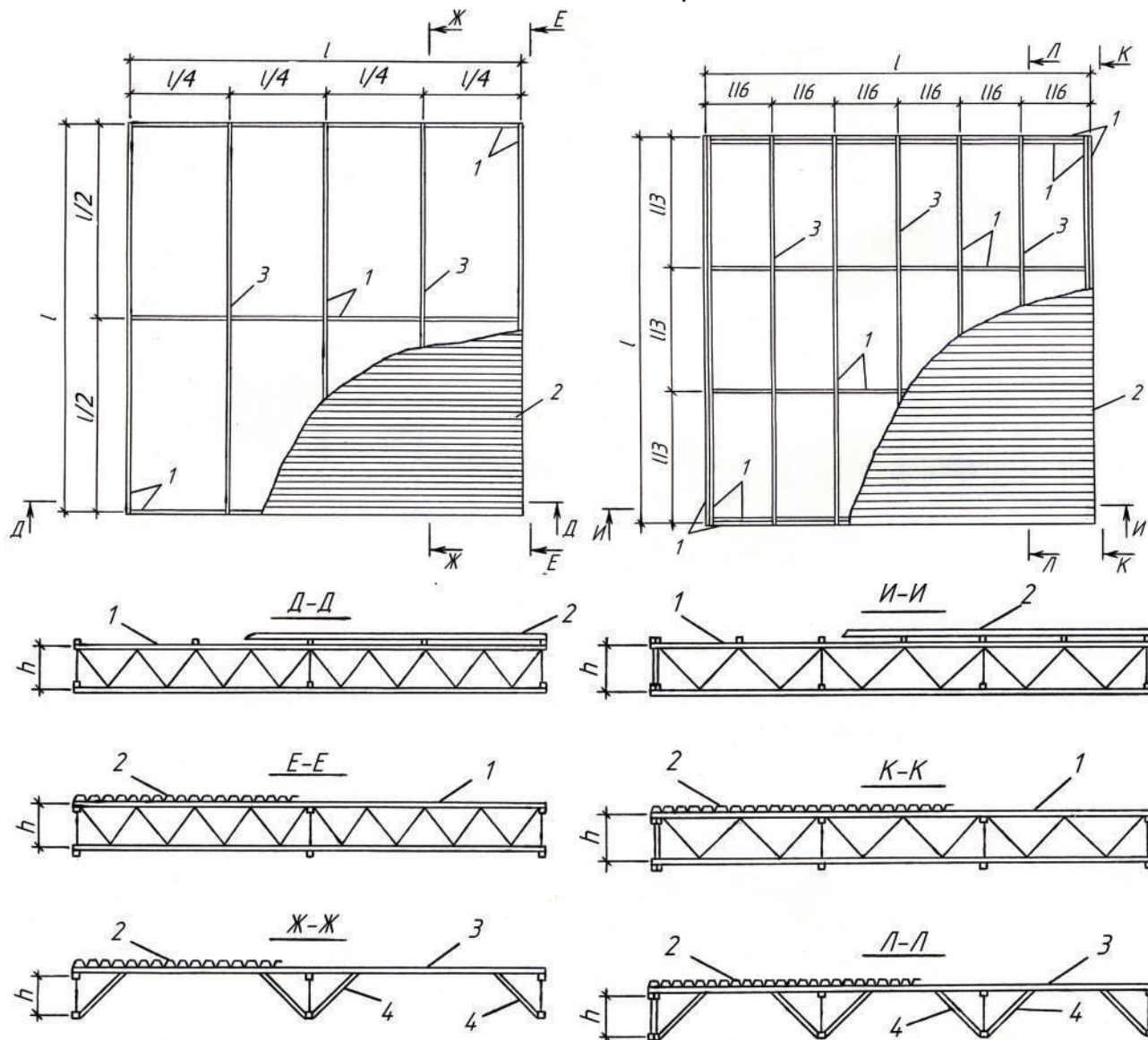
Рис. 3. Схемы модуля типа «Пятигорск» из перекрестных ферм с прогонами при количестве ячеек 2 \times 2 (а) и 3 \times 3 (б): 1 – одиночные перекрестные фермы; 2 – элементы ограждения (профилированные листы); 3 – прогоны; 4 – подкосные элементы
