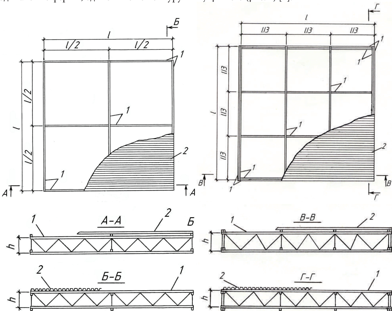
Рис. 2. Схемы модуля типа «Пятигорск» из перекрестных ферм при количестве ячеек 2 \times 2 (а) и 3 \times 3 (б): 1 – одиночные перекрестные фермы; 2 – элементы ограждения (профилированные листы)
