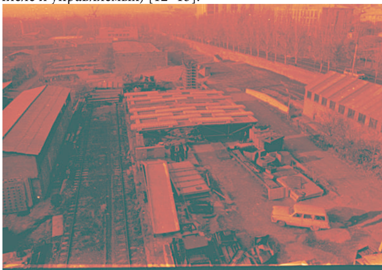
Рис. 5. Общий вид испытательного полигона АрмНИИСА с опытно-промышленным образцом блока покрытия (на переднем плане) и моделью 9-этажного каркасного здания с динамическим гасителем колебаний в виде гибкого верхнего этажа (на заднем плане)
