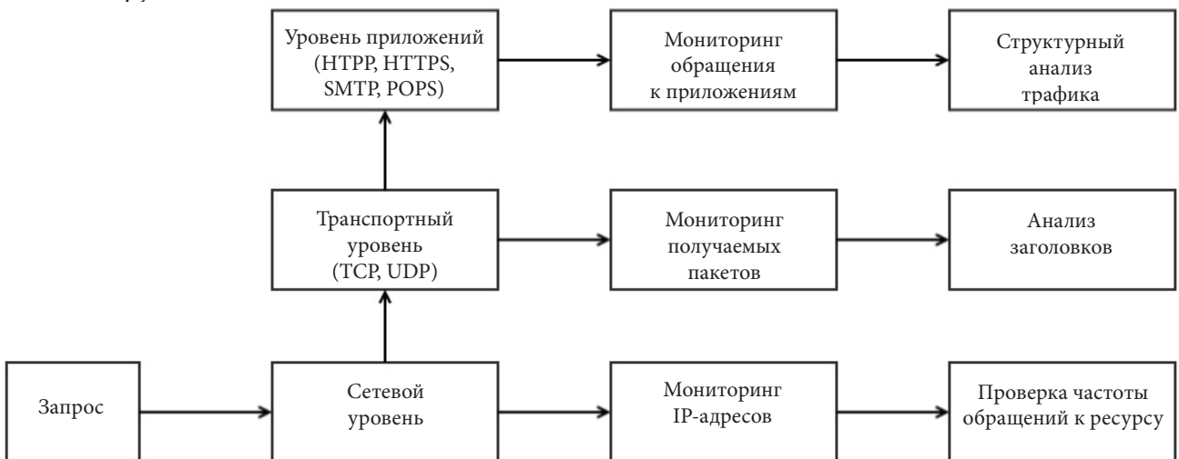
Рис. 1. Схема мониторинга получаемого запроса на предмет выявления DDOS-атаки
