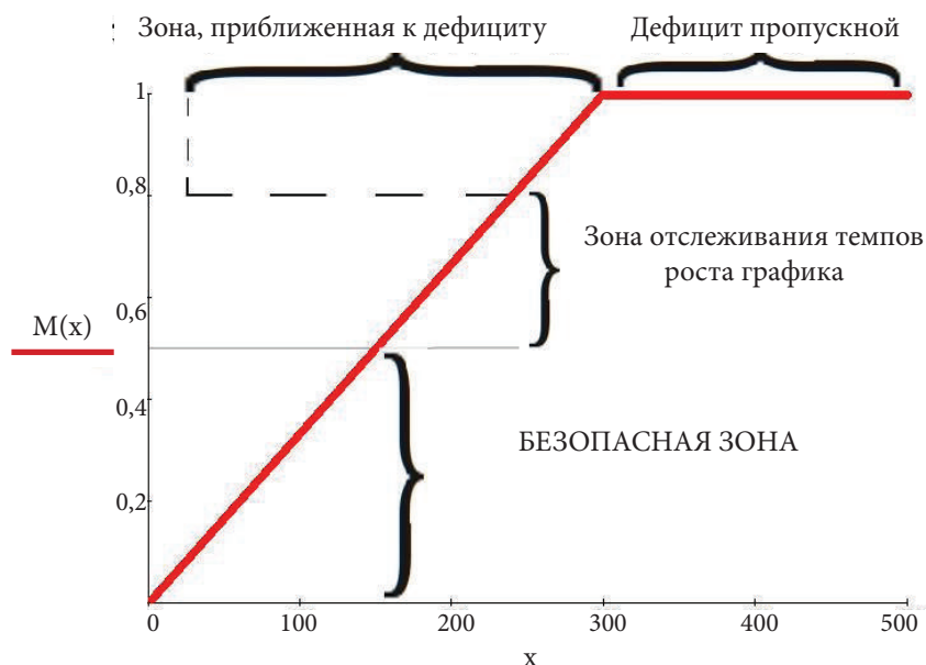
Рис. 2. Оценка загрузки канала
