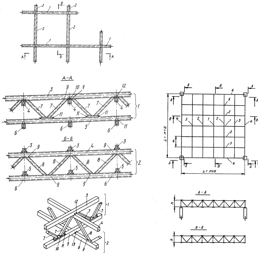
Рис. 1. Схемы перекрестных ферм:
